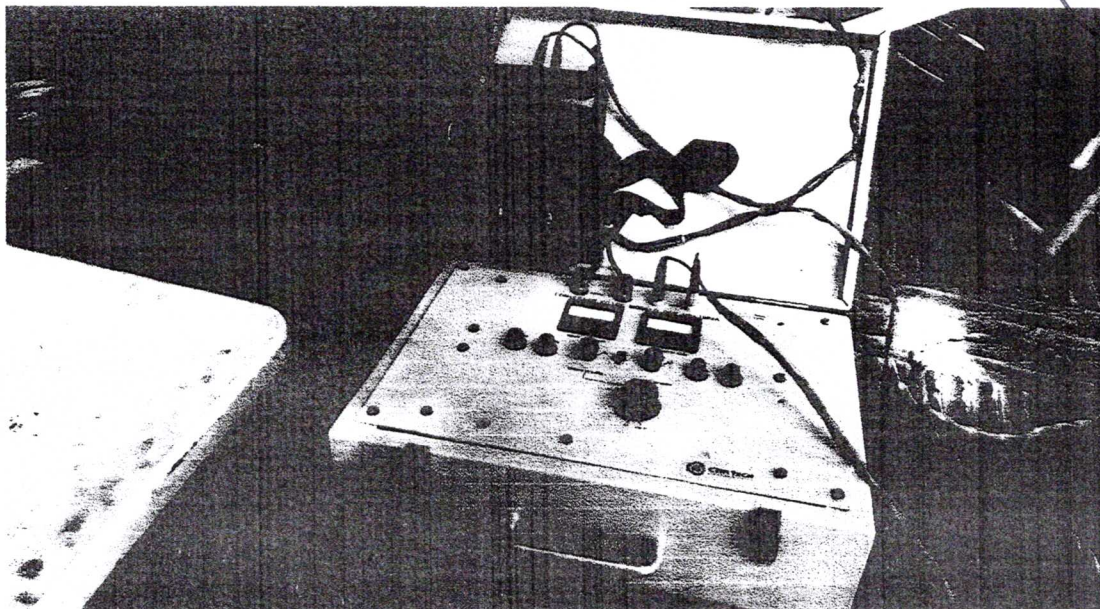
Equipamento utilizado para a aquisição dos dados geofísicos - Eletroresistivímetro CC/CC modelo CDC 1000/12R2A da CTRLTECH.
